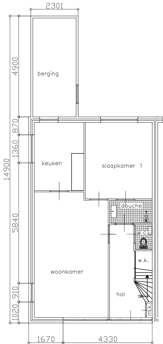
PLATTEGROND.
